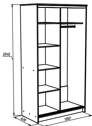
корпус 2-х дверного шкафа*
